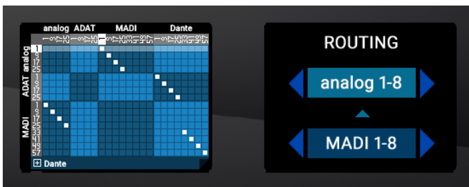
ROUTING MENU A32pro Dante
